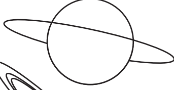
URANUS
